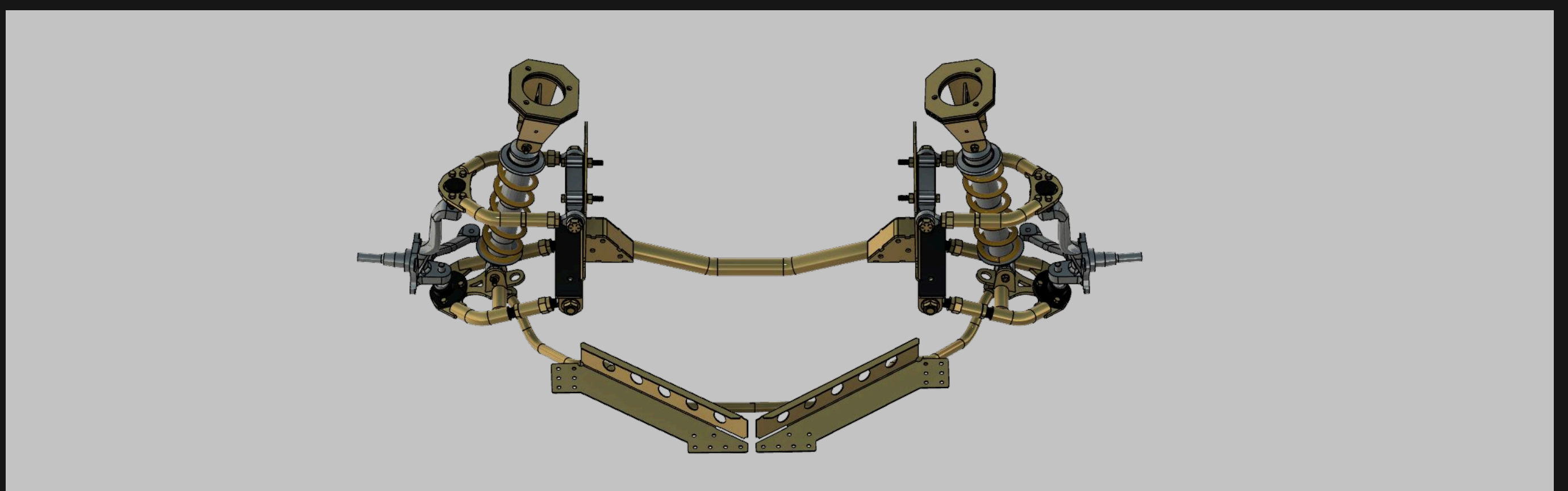
ZAWIESZENIE PRZEDNIE WIELOWAHACZOWE FORD MUSTANG 1964/5-1968 OHLINS
